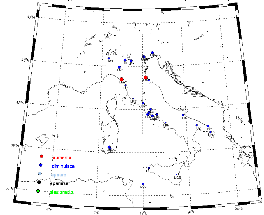
NOV - Rapporto tra le % di occorrenza di vento < 5 nodi [2000-09/1980-89]
