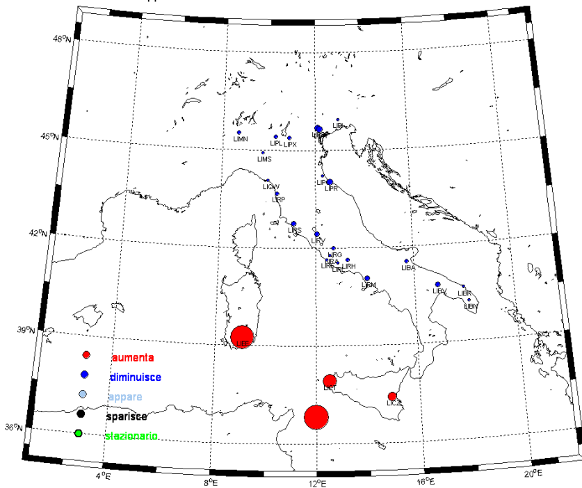
OTT - Rapporto tra le % di occorrenza di visibilità < 1000mt. 2000-09/1980-89
