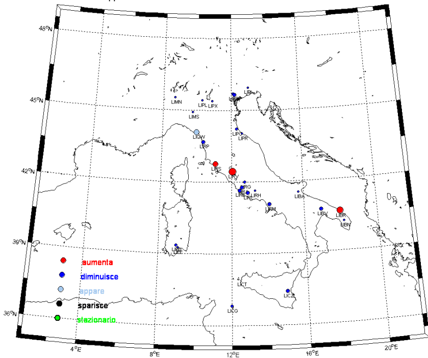
NOV - Rapporto tra le % di occorrenza di visibilità < 1000mt. 2000-09/1980-89
