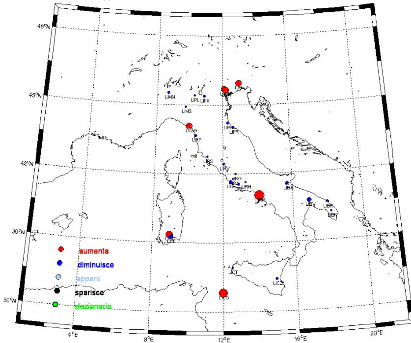
FEB - Rapporto tra le % di occorrenza di visibilità < 1000mt. 2000-09/1980-89
