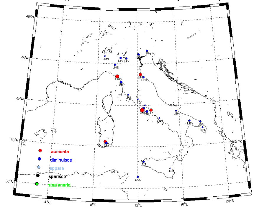
SET - Rapporto tra le % di occorrenza di vento < 5 nodi [2000-09/1980-89]
