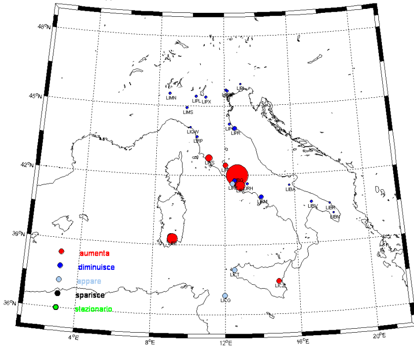
GEN - Rapporto tra le % di occorrenza di visibilità < 1000mt. 2000-09/1980-89
