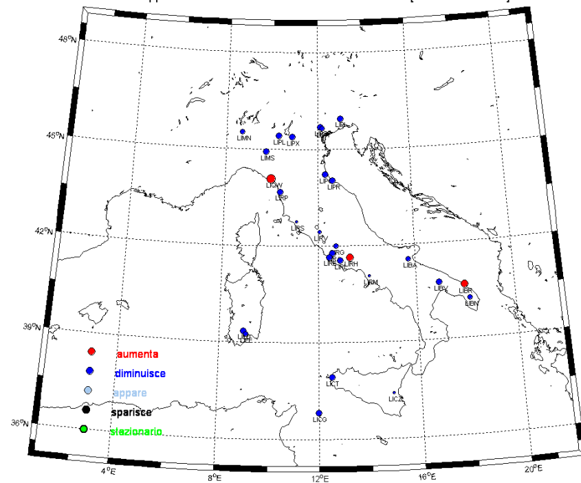
DIC - Rapporto tra le % di occorrenza di vento < 5 nodi [2000-09/1980-89]
