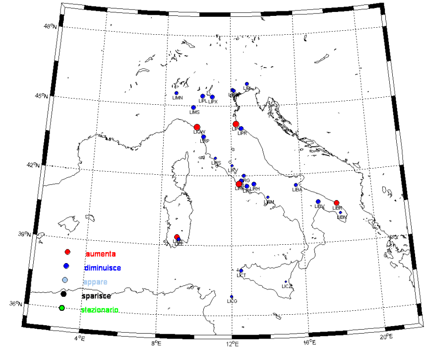
MAR - Rapporto tra le % di occorrenza di vento < 5 nodi [2000-09/1980-89]
