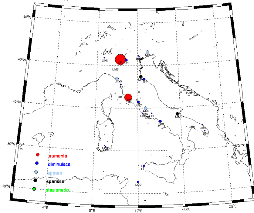
LUG - Rapporto tra le % di occorrenza di visibilità < 1000mt. 2000-09/1980-89
