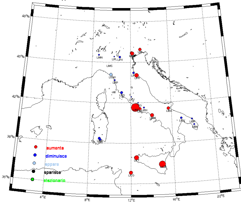
MAG - Rapporto tra le % di occorrenza di visibilità < 1000mt. 2000-09/1980-89
