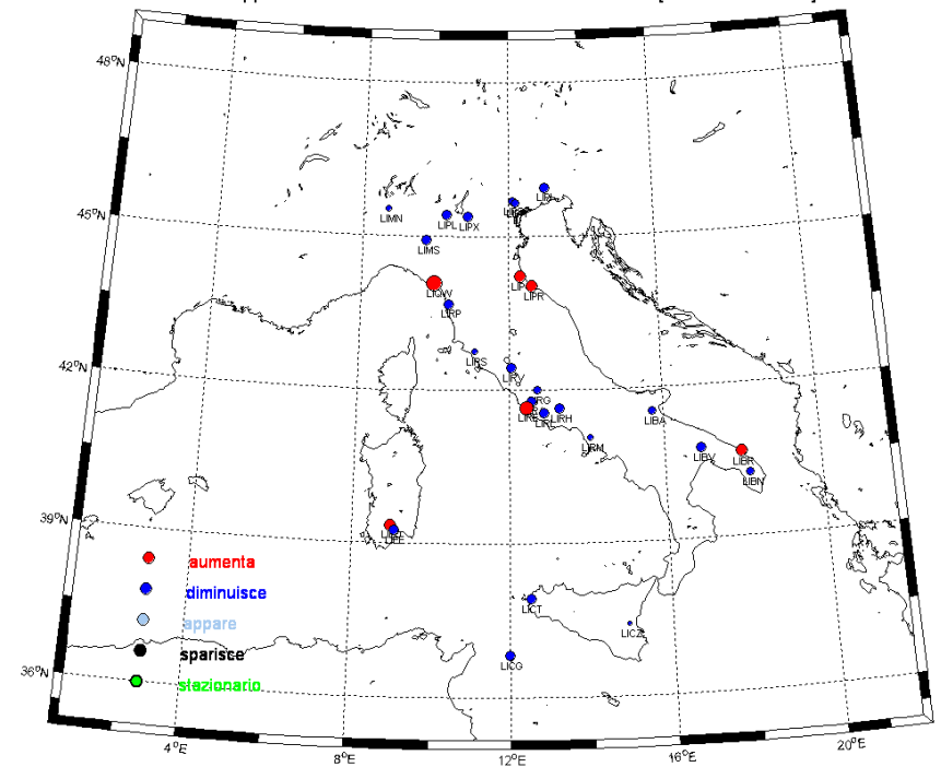
OTT - Rapporto tra le % di occorrenza di vento < 5 nodi [2000-09/1980-89]
