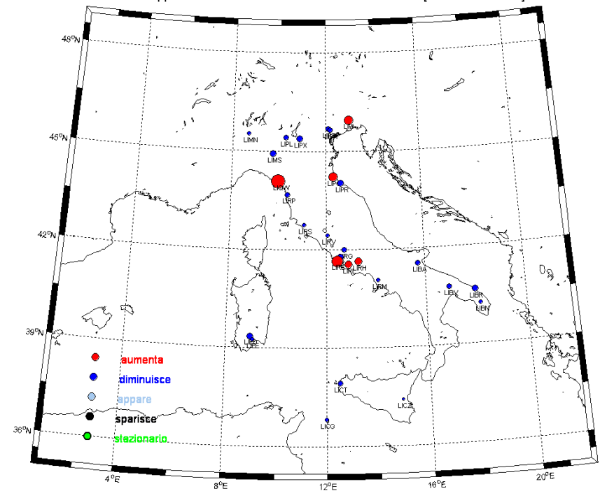
MAG - Rapporto tra le % di occorrenza di vento < 5 nodi [2000-09/1980-89]
