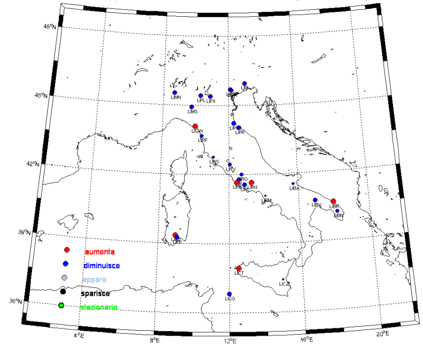
GEN - Rapporto tra le % di occorrenza di vento < 5 nodi [2000-09/1980-89]
