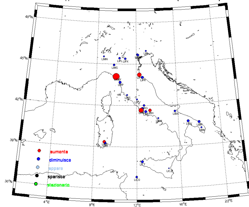
AGO - Rapporto tra le % di occorrenza di vento < 5 nodi [2000-09/1980-89]
