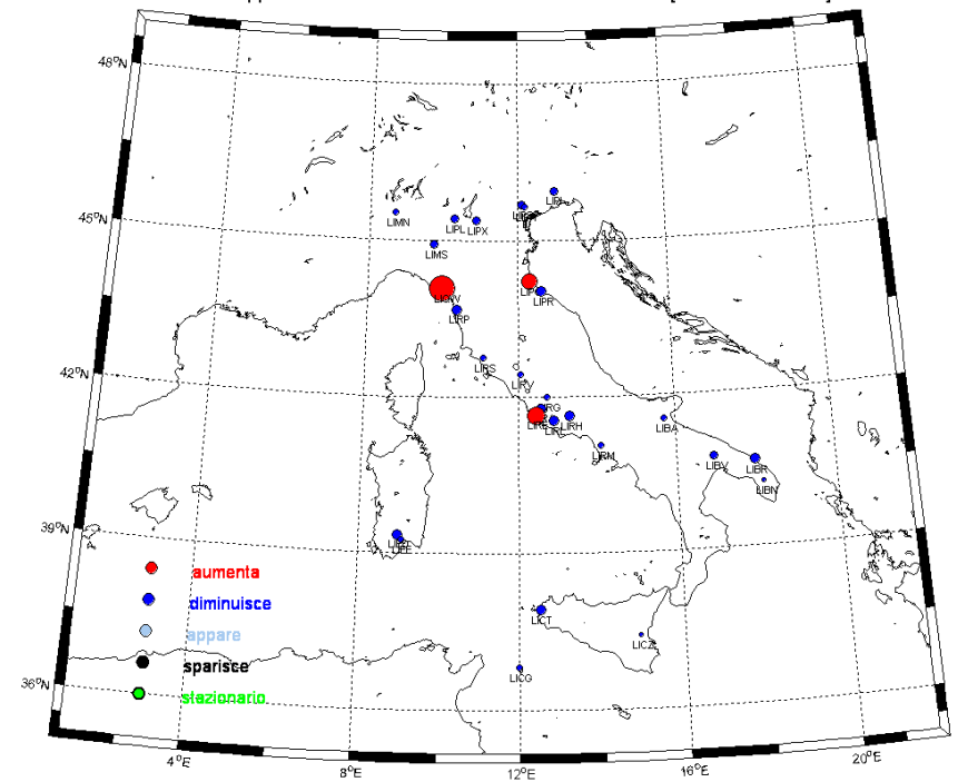
LUG - Rapporto tra le % di occorrenza di vento < 5 nodi [2000-09/1980-89]
