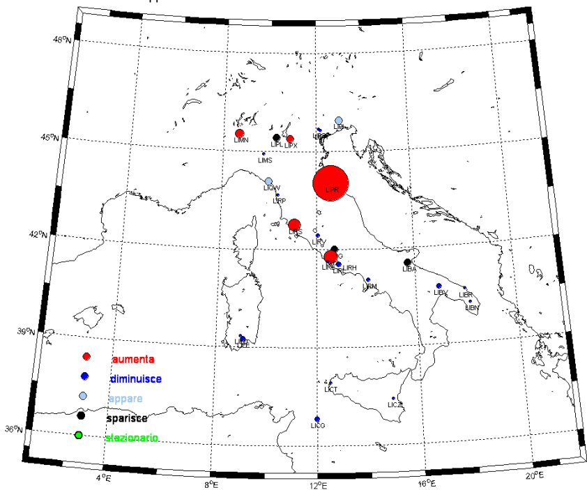
AGO - Rapporto tra le % di occorrenza di visibilità < 1000mt. 2000-09/1980-89
