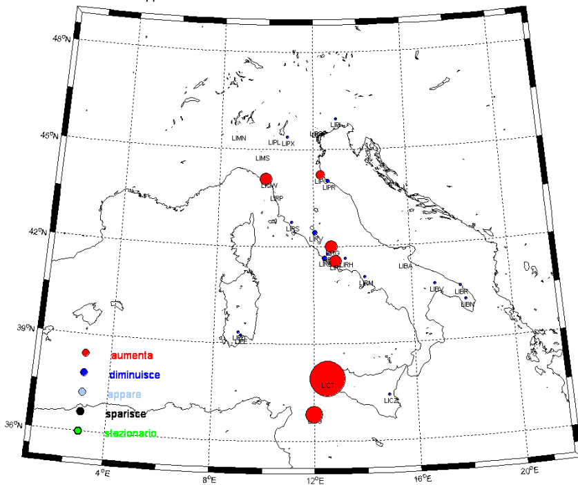
SET - Rapporto tra le % di occorrenza di visibilità < 1000mt. 2000-09/1980-89
