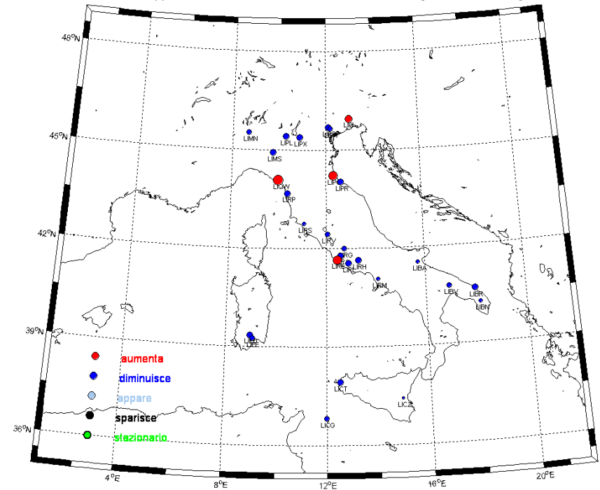
FEB - Rapporto tra le % di occorrenza di vento < 5 nodi [2000-09/1980-89]
