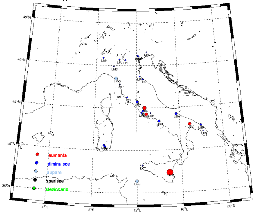
DIC - Rapporto tra le % di occorrenza di visibilità < 1000mt. 2000-09/1980-89
