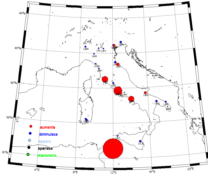
MAR - Rapporto tra le % di occorrenza di visibilità < 1000mt. 2000-09/1980-89
