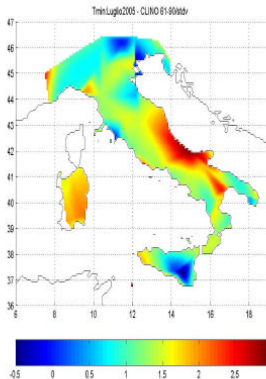
Anomalie delle temperature minime del mese di Luglio 2005 confrontate con la climatologia
