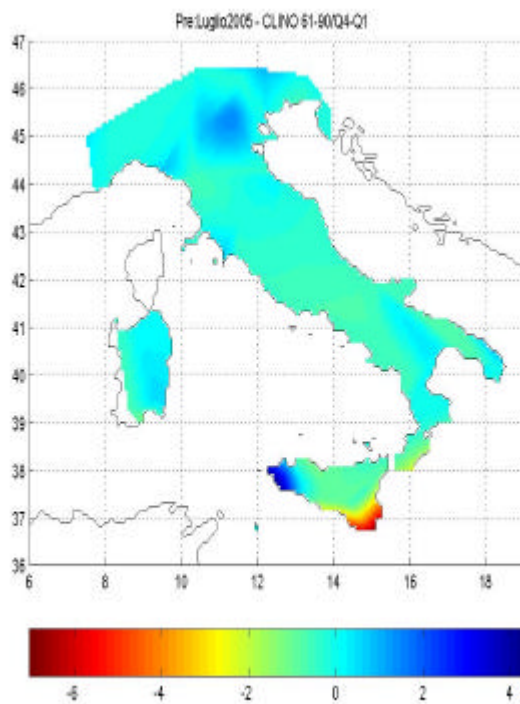
Anomalie delle precipitazioni cumulate del mese di Luglio 2005 confrontate con la climatologia
