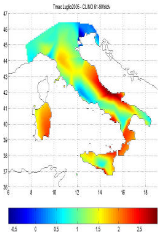
Anomalie delle temperature massime del mese di Luglio 2005 confrontate con la climatologia
